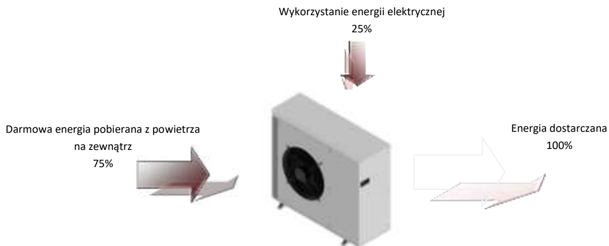
Rysunek 2.2. Działanie aerotermalnej pompy ciepła w normalnych warunkach.
